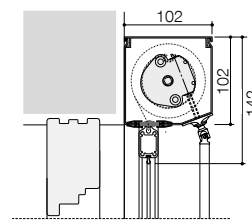
Kurbelantrieb
