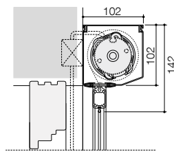
Motorantrieb
